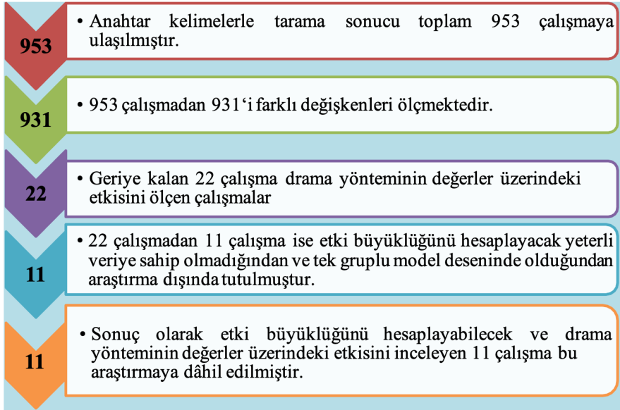
Şekil 1. Akış Diyagramı
